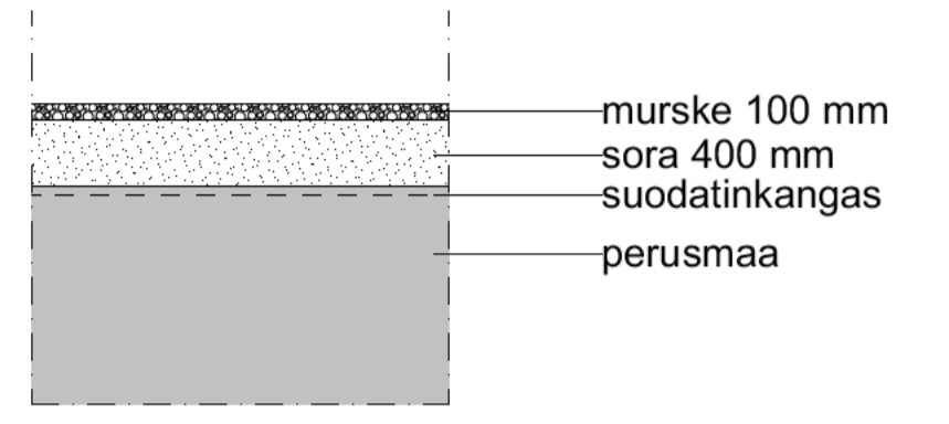
murskepihan rak.leikkaus (1:50)
