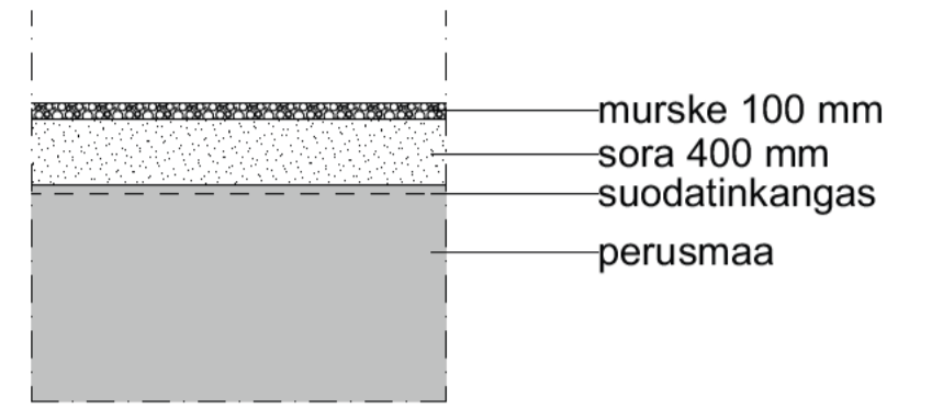
murskepihan rak.leikkaus (1:50)
